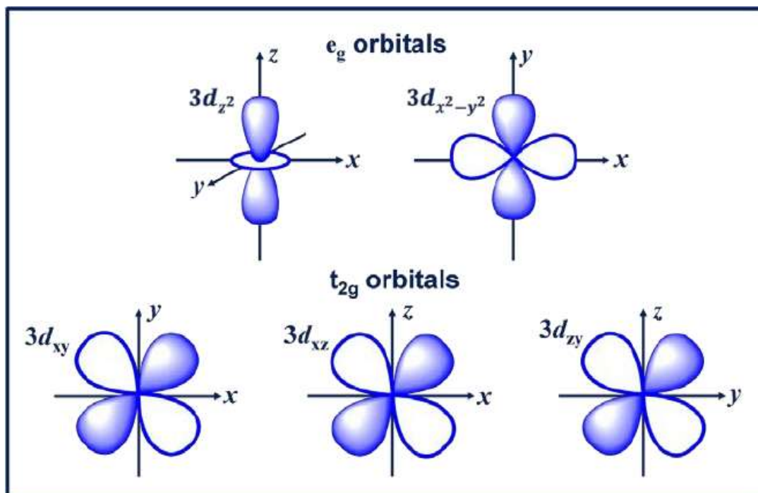
Fig: Grouping of d-orbitals
